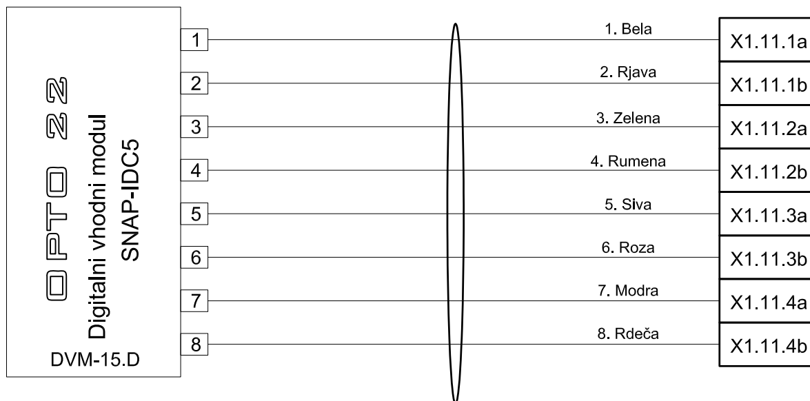
Kabel LiYY 16x0.25mm
