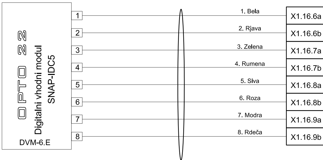
Kabel LiYY 16x0.25mm
